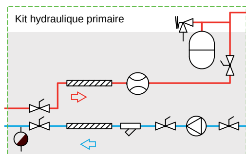
Circulateur intégré
