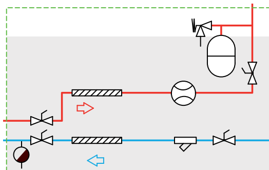
Sans circulateur
